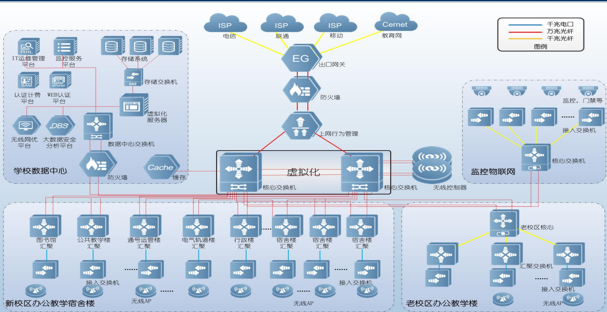
湖南铁道职业技术学院网络拓扑图
